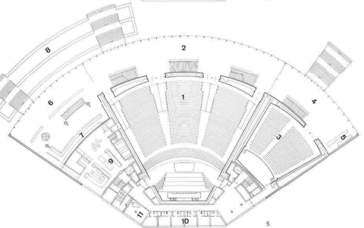
5 Grundriß Saalgeschoß 1:800. Plan au niveau de la salle. Plan of hall level.
